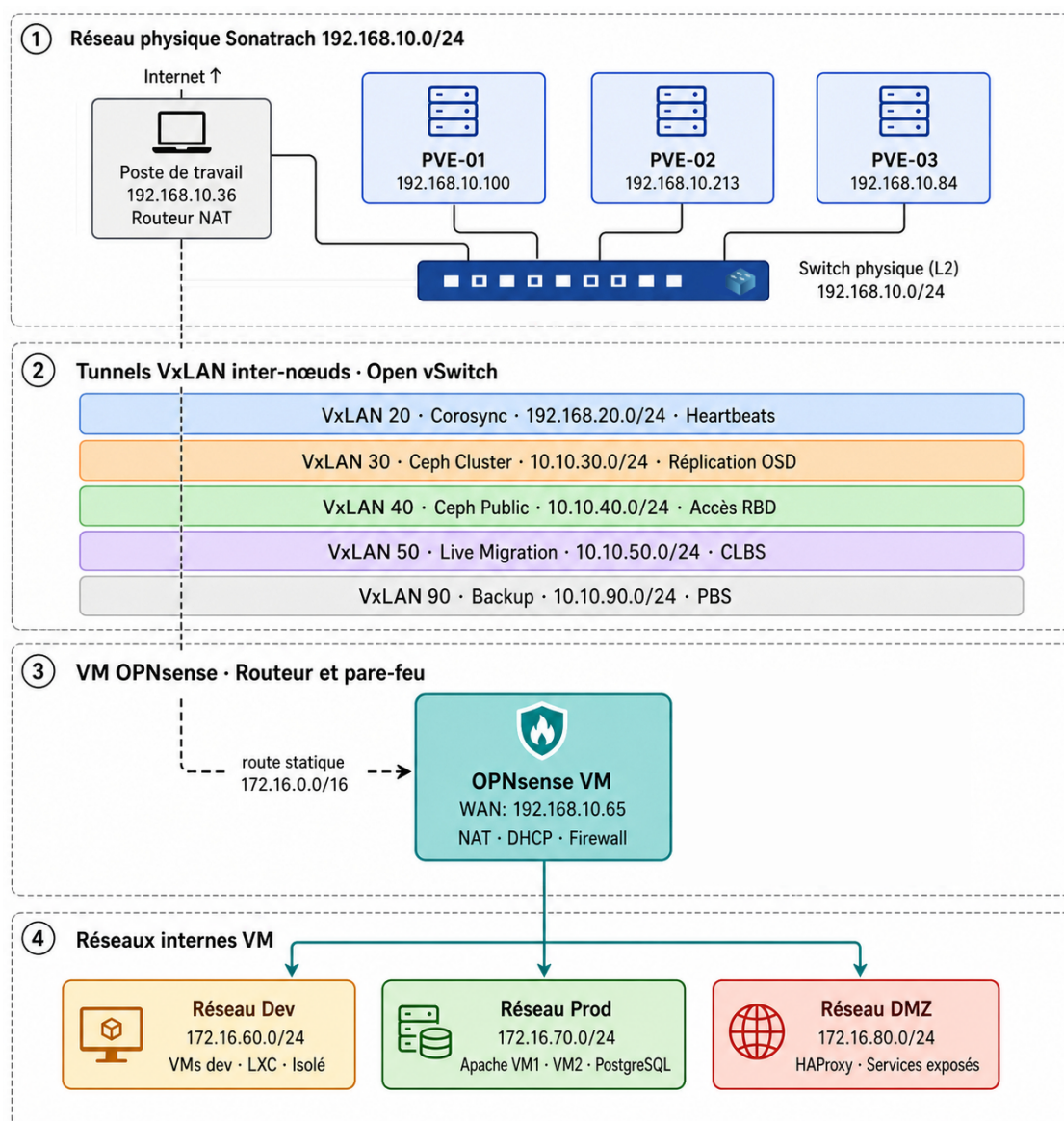
FIGURE III.4 – Topologie Réseau et Plan VxLAN
